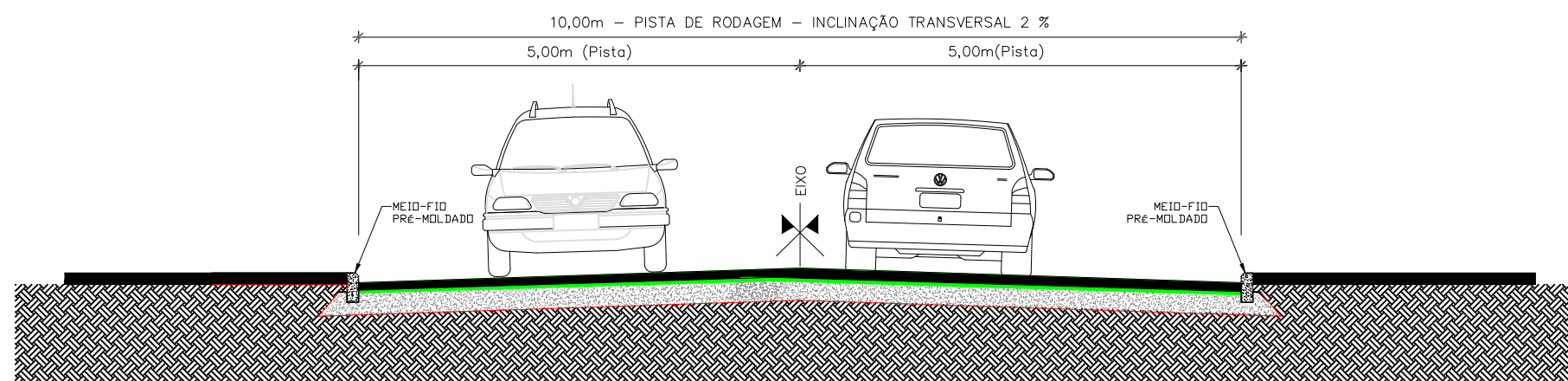
SEÇÃO TIPO DE PAVIMENTAÇÃO ASFÁLTICA - RUA JOSÉ SEVERINO PICK E CHARLOTTE MANDLER
